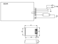
Technische Daten Philips HID-PV C 35 /S CDM 220-240V 50/60Hz für 35W
